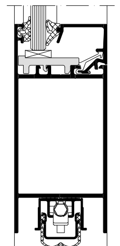
Schüco Tür ADS 50.NI, Maßstab 1:2 Schüco Door ADS 50.NI, scale 1:2
